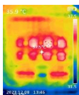
ภายในตู้ DC Panel Box อุณหภูมิ 37.5 °C
