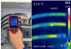
สาย MCCB 37.8 °C
