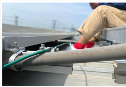
Torque screw ขนาด 13 mm. และขนาด 17 mm.
