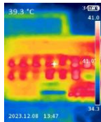
ภายในตู้ DC Panel Box อุณหภูมิ 41.0 °C
